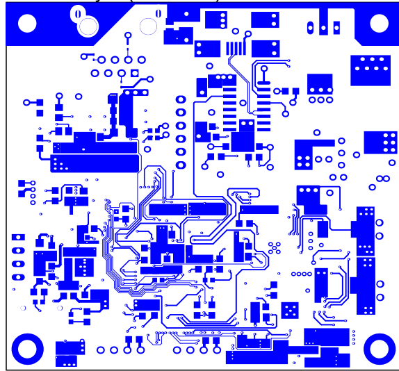
Bottom Layer (Scale 1:1)
